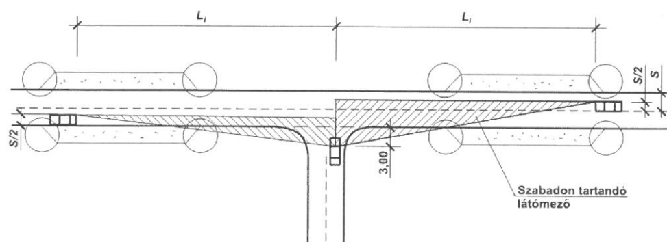
1.15. ábra – Elindulási látómező ( L_1 – elindulási látótávolság)
